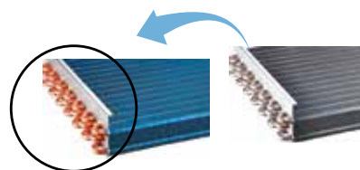
Alhetas hidrófilas + tubagem de interior rosca
