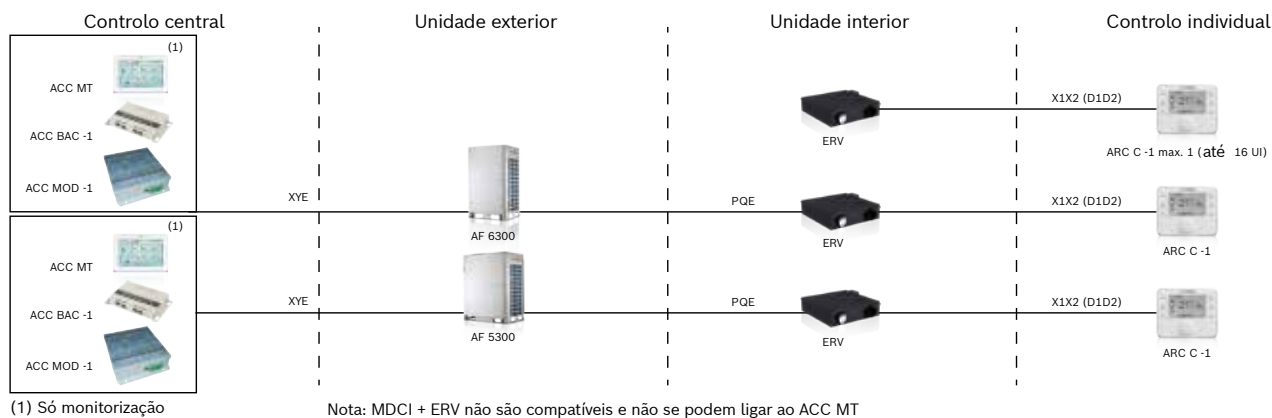
Diagrama das unidades de ventilação ERV
