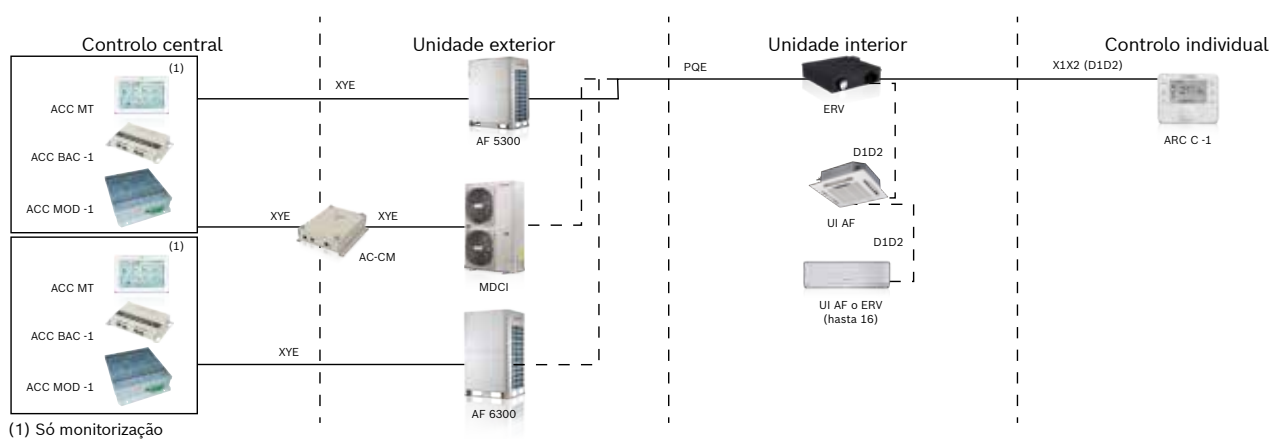
Diagrama das unidades de ventilação ERV com unidades interiores
